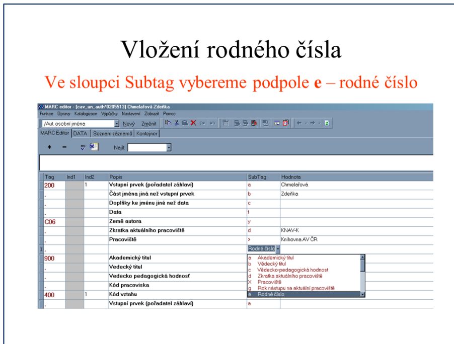
Obr. 11. Výběr podpole pro rodné číslo
